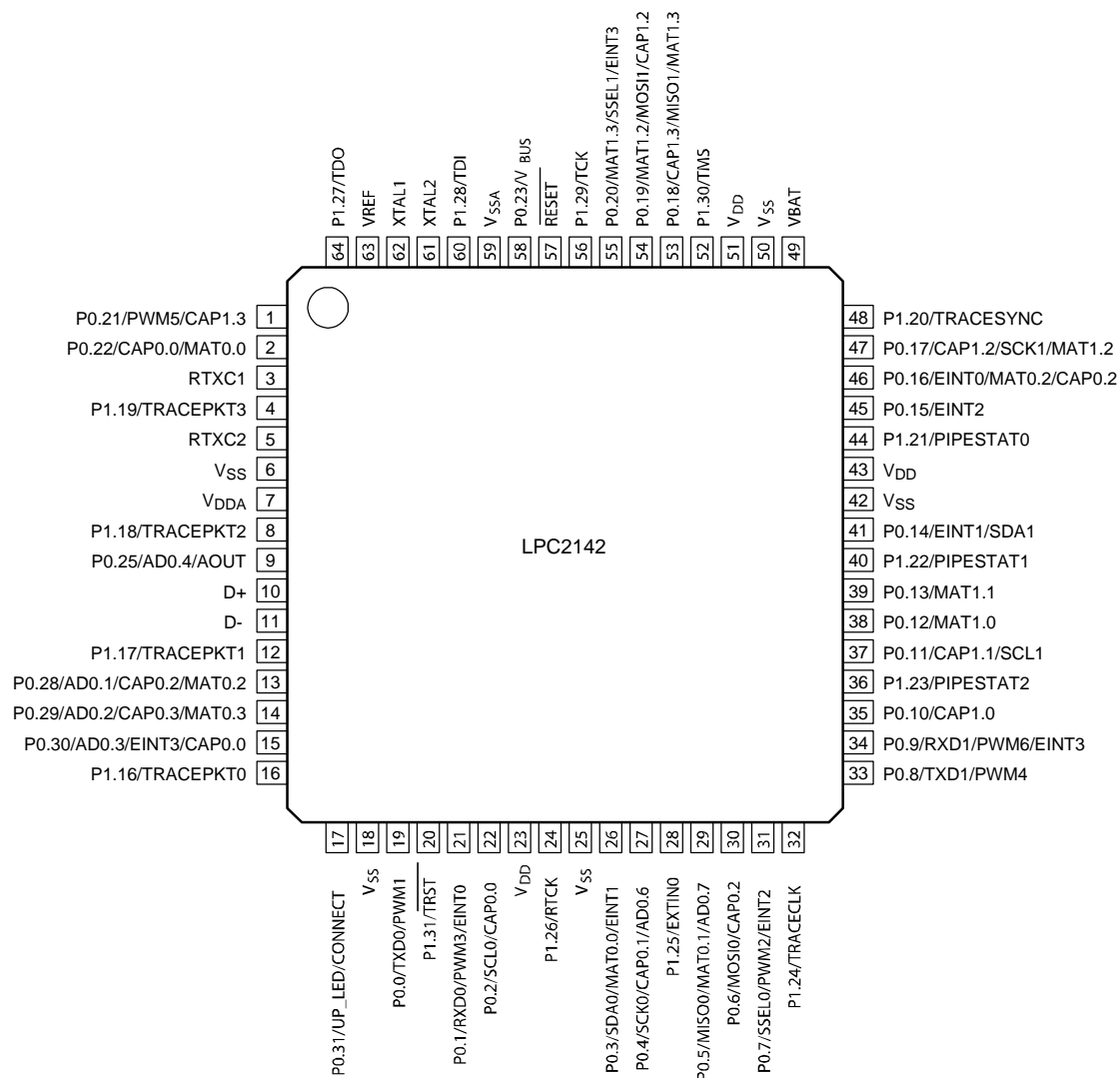
图3 LPC2142 管脚配置
