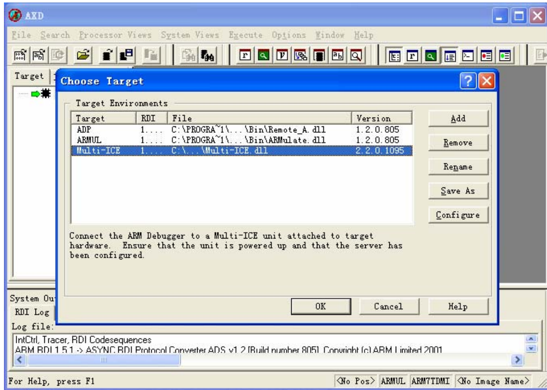
选择 MultiICE.dll 图
